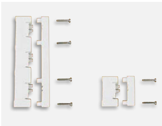
1 og 3 póla safnskinnuhöldur fyrir 12 x 5, 12 x 10, 20 x 5, 20 x 10, 30 x 5 og 30 x 10 mm safnskinnur úr kopar
